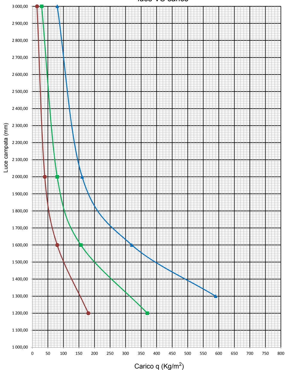
luce VS carico
