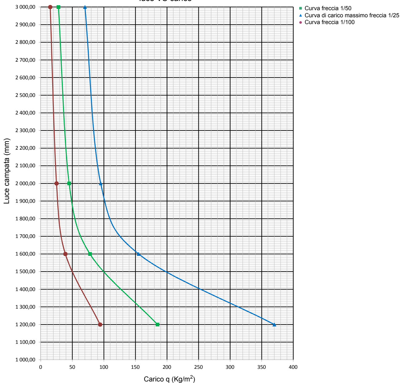
luce VS carico
